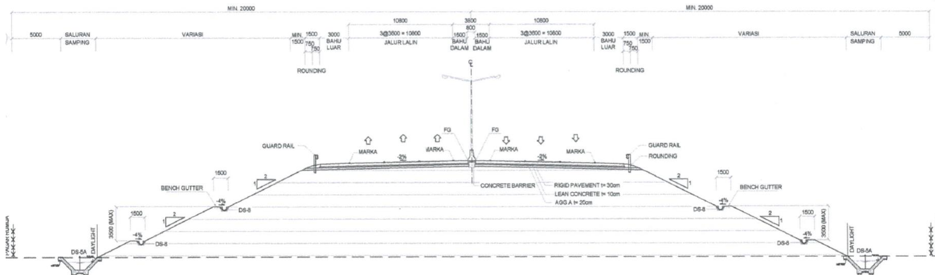
TIPIKAL POTONGAN MELINTANG JALAN UTAMA DAERAH TIMUNAN
